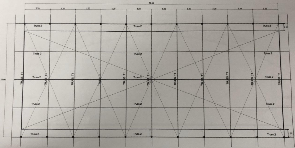
แปลน โครงสร้างหลังคา Scale 1 : 150
