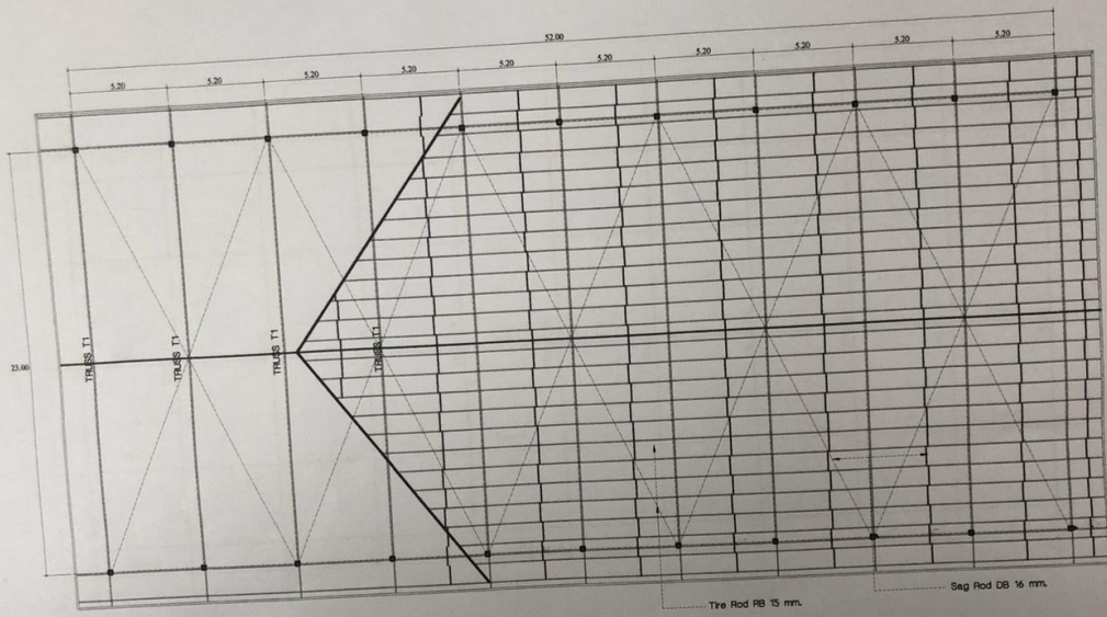
แปลนโครงสร้างหลังคา Scale 1 : 100
