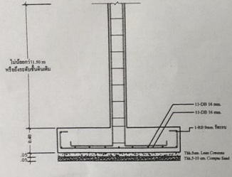
Detail F1 (Section)
